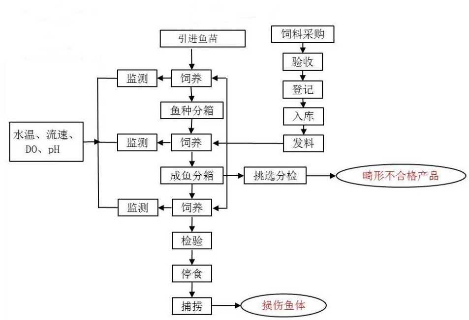
图 2-1 项目主要工艺流程及产污位置图
